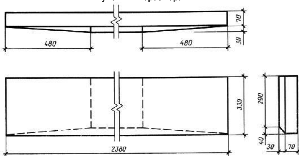
Ступени типоразмера ЛСС24
