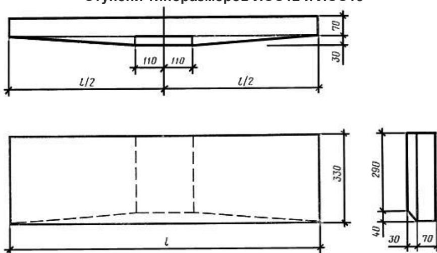
Ступени типоразмеров ЛСС12 и ЛСС15
